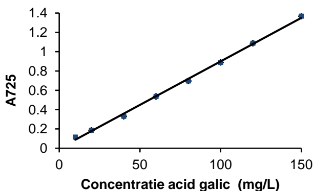
Figura 1. Curba de calibrare absorbantă vs. concentrația acidului galic.
