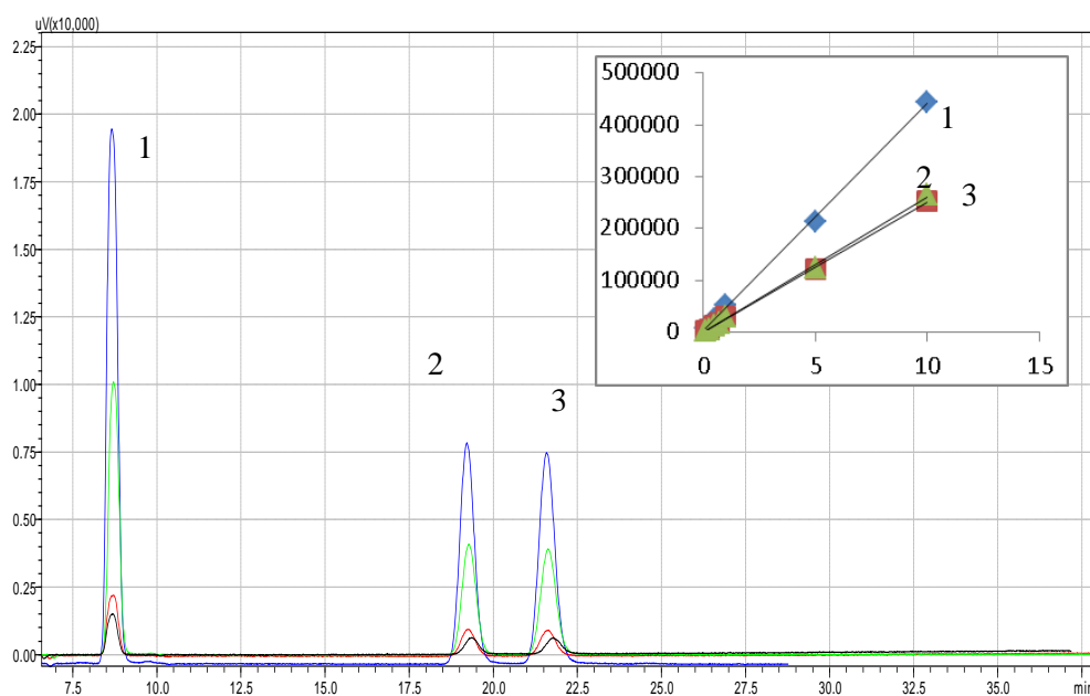
Figura 2. Cromatogramele HPLC-DAD suprapuse pentru 4 concentrații (0,7; 1; 5; 10 \mu\text{g/mL} ) de silicristin (1), silibinin A (2) și silibinin B (3); inset dreptele de etalonare
