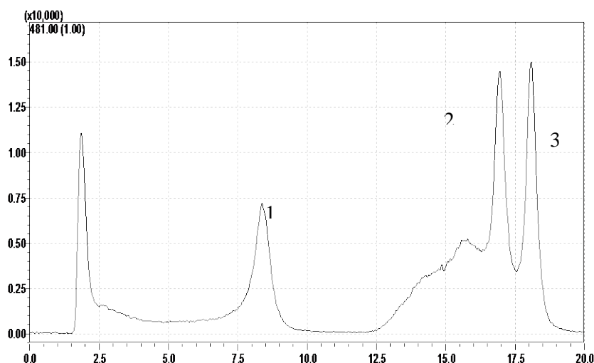
Figura 3. Cromatogramele HPLC-MS obținute pentru amestecul de standarde (1- silicristin, 2-silibinin A, 3-silibinin B; concentrație 0,5 \mu\text{g}/\text{mL} ).
